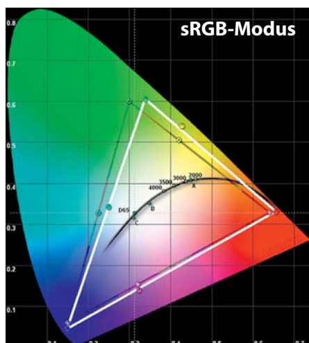
Im sRGB-Modus deckt der SX7 den sRGB-Referenzfarbraum (dunkles Dreieck) zwar nicht ganz ab, aber er trifft ihn besser als der SX60.
