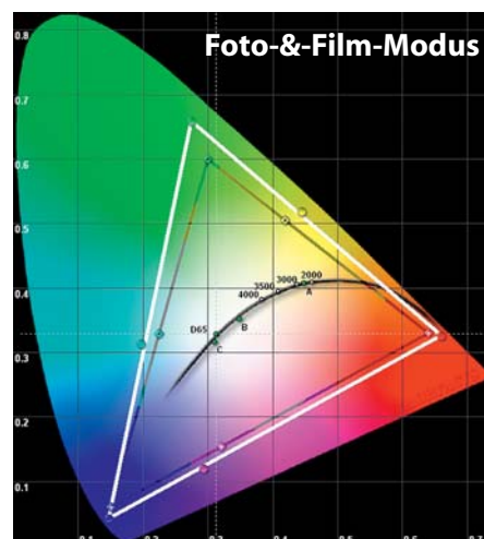
Der Foto-&Film-Modus besitzt einen sehr großen Farbraum. Deutliche Verbesserungen gibt es im Tonwertbereich von Cyan und Grün.
