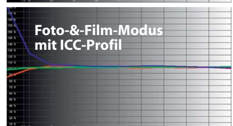
Der Foto-&Film-Modus ist mit 7.241 Kelvin etwas zu blau. Mit einer Kalibrierung und einem ICC-Profil lässt sich der SX7 auf 6.500 Kelvin optimieren.
